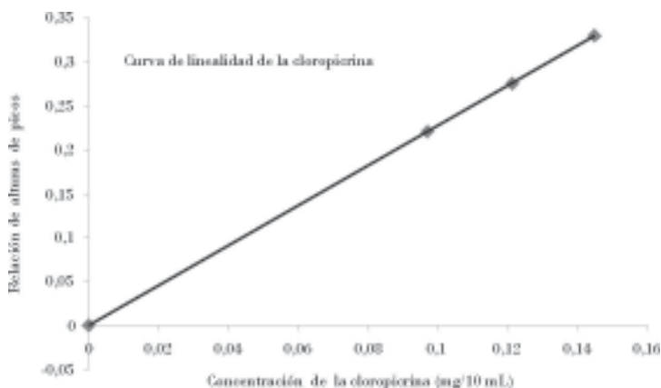
Figura 2. Curva de calibración en la determinación de la cloropirina.
