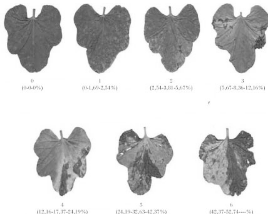
Figura 1. Escala logarítmica diagramática para evaluar severidad del mildiú de las cucurbitáceas en el patosistema Pseudoperonospora-Cucumis melo .
