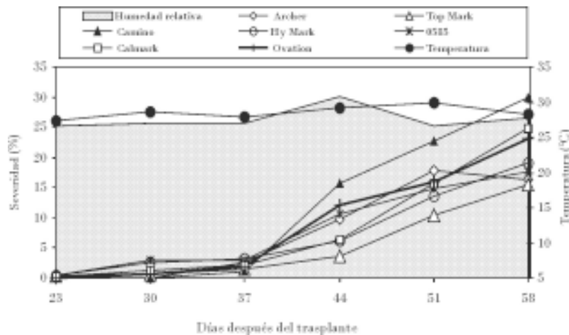
Figura 2. Curvas del progreso de la enfermedad de materiales de melón en el patosistema Pseudoperonospora cubensis - Cucumis melo de los 23 a los 58 ddt .
